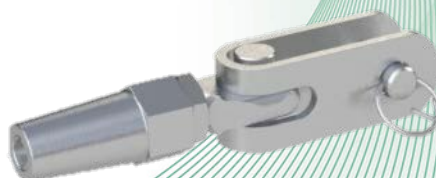
Bild 6: Endverbinder verschraubt
