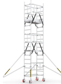
ABS Ein-Personen-Arbeitsbühne
