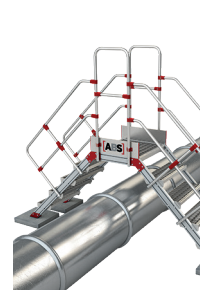
ABS Überstieg
