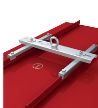
ABS-Lock® Falz IV Stehfalz
