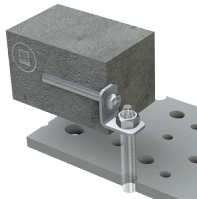
Winkel zur seitlichen Befestigung
