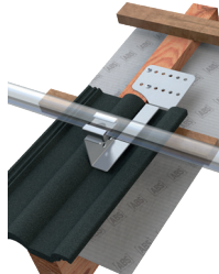
ABS AluTrax Steildach Halter
