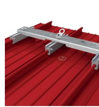
ABS-Lock® Falz VI Rundbördelfalz
